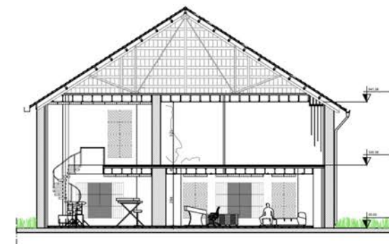
DD KESİTİ
