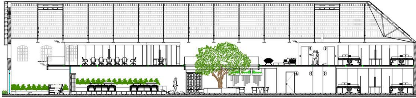
1/50 ÖLÇEK K1 KESİTİ
