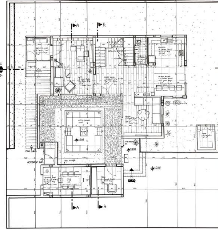
EĞİN KAT PLANI ÖLÇEK 1/50
