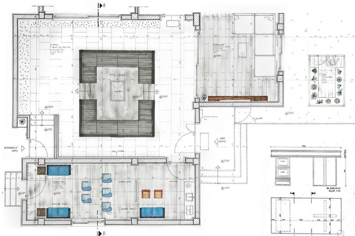
4. KAT PLANI ÖLÇEK 1/50
