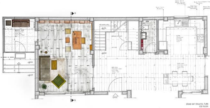
2. KAT PLANI ÖLÇEK 1/50
