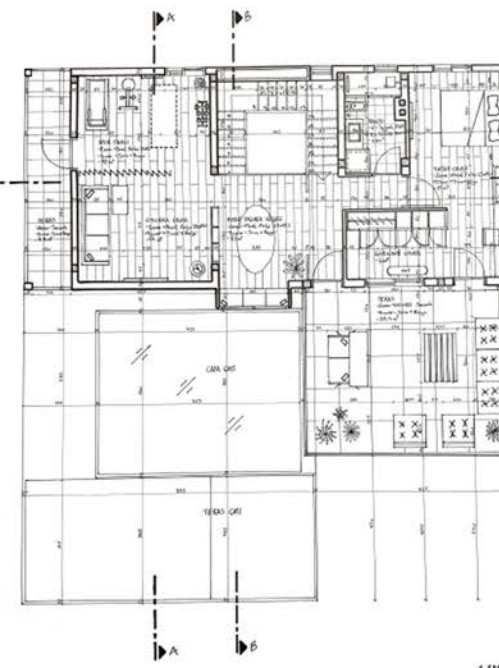
1. KAT PLANI ÖLÇEK 1/50
